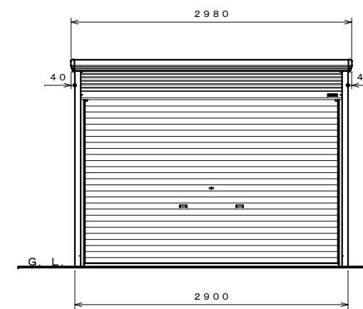
正面図 S=1:40
