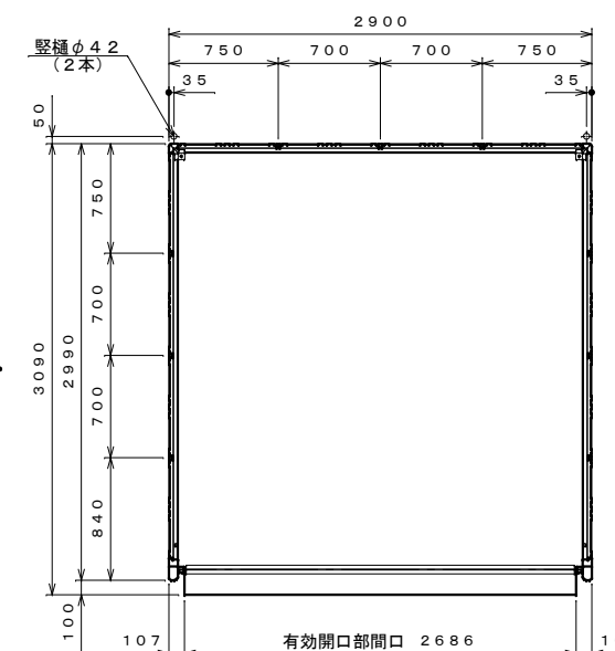
平面図 S=1:40
