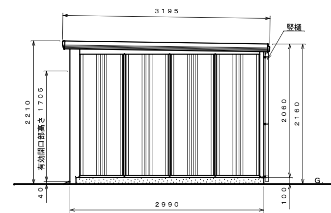
側面図 S=1:40
