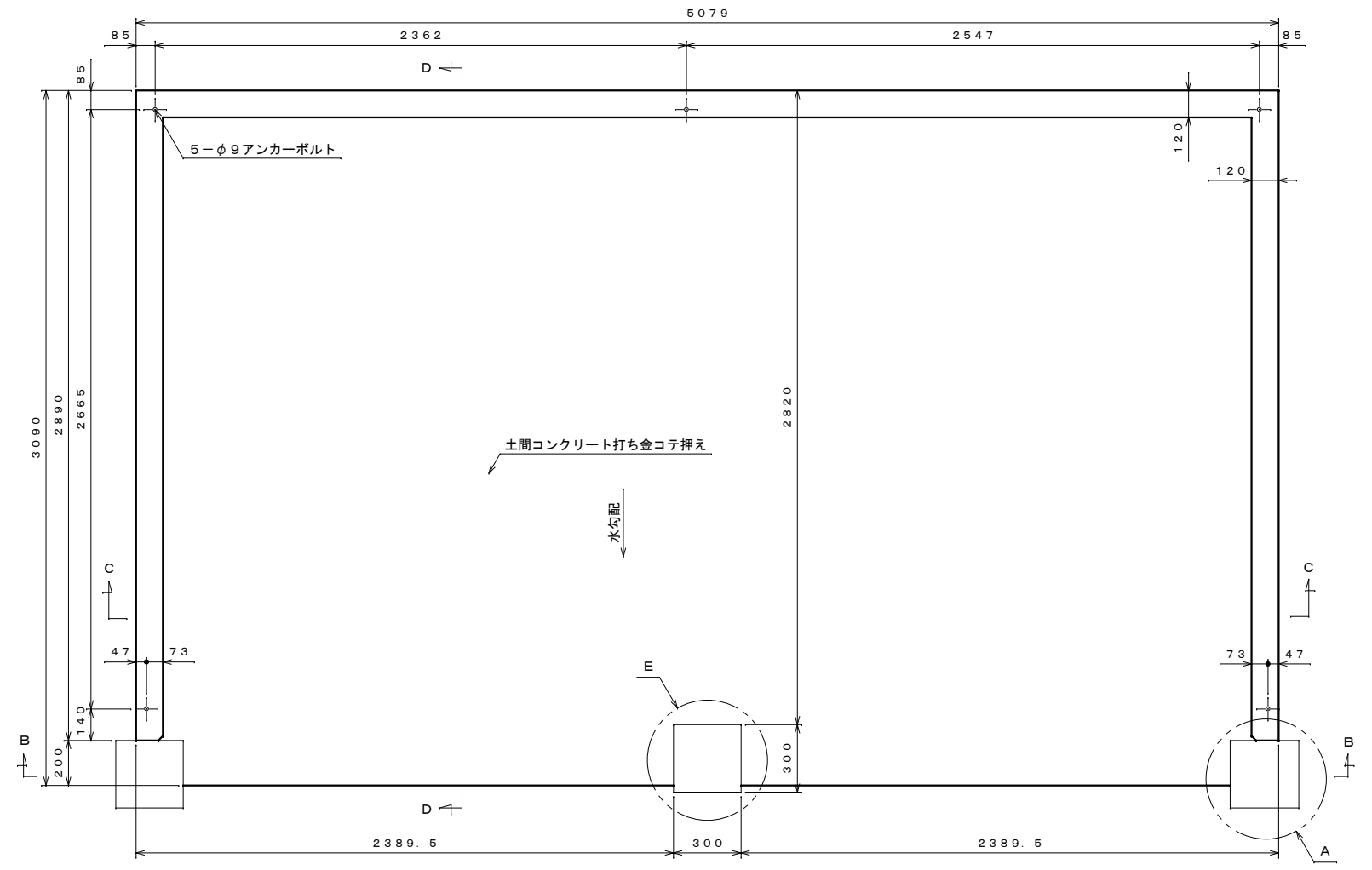
基礎伏せ図 S=1:20 【注：この基礎は標準を示しています。現場の実情に合わせて、ご設計下さい。】
