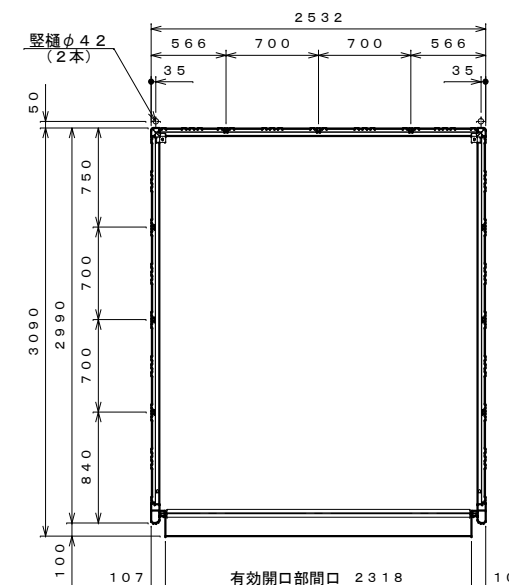
平面図 S=1:40
