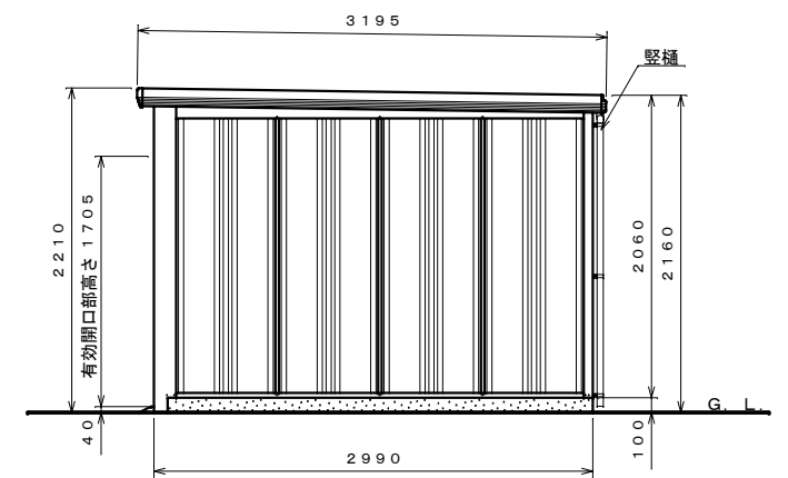
側面図 S=1:40
