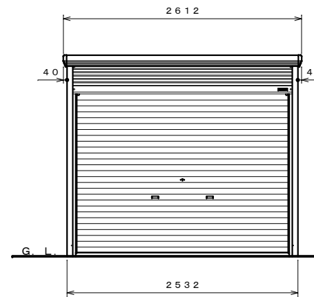
正面図 S=1:40
