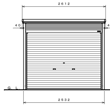
正面図 S=1:40
