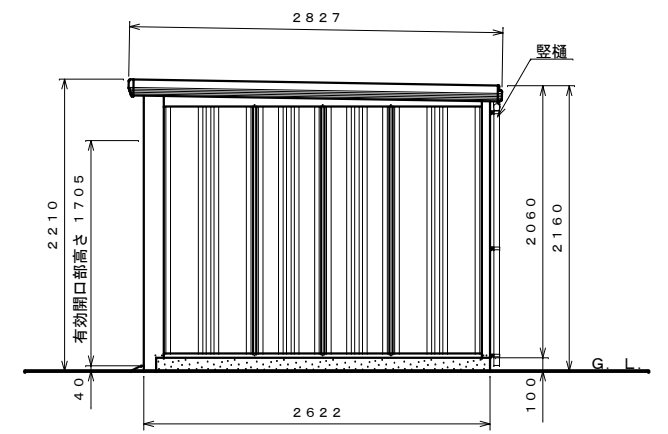
側面図 S=1:40
