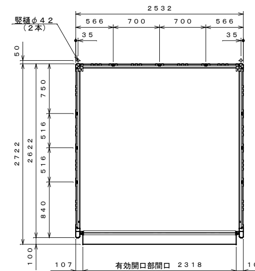
平面図 S=1:40
