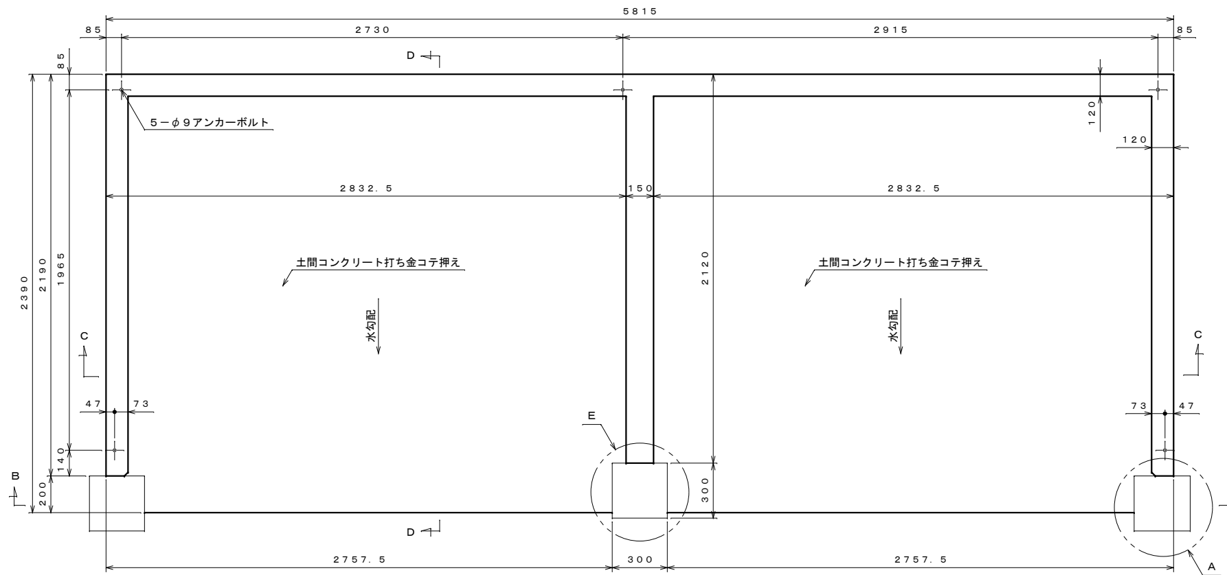
基礎伏せ図 S=1:20
