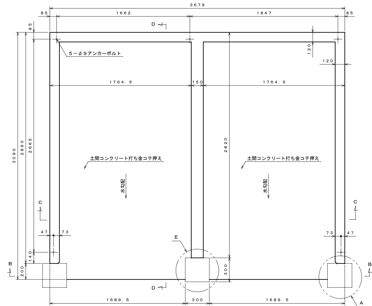
基礎伏せ図 S=1:20
