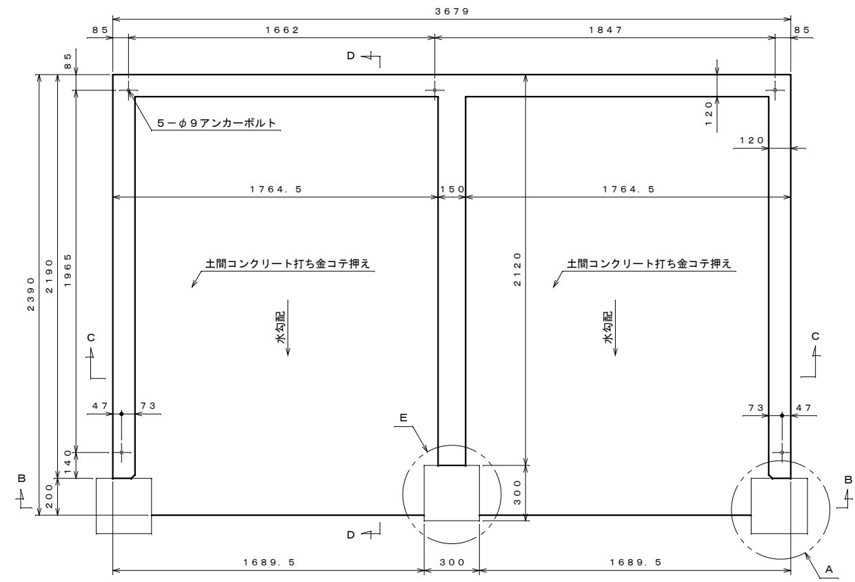
基礎伏せ図 S=1:20
