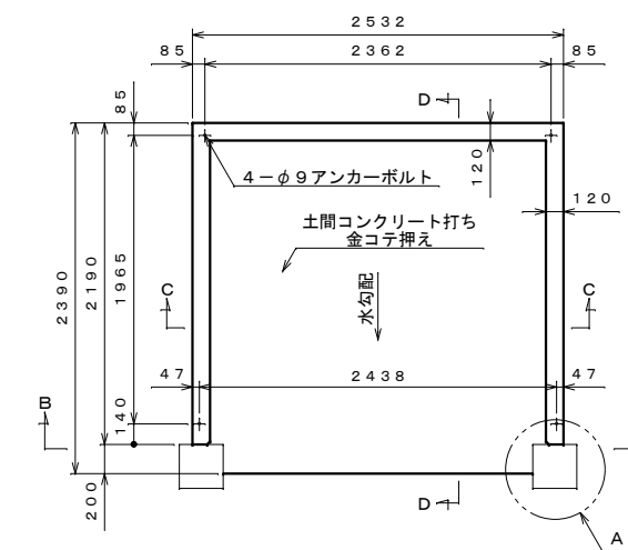
基礎伏せ図 S=1:40
