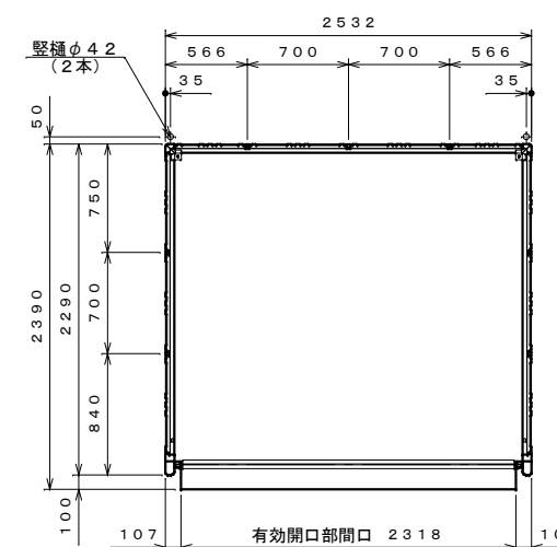
平面図 S=1:40
