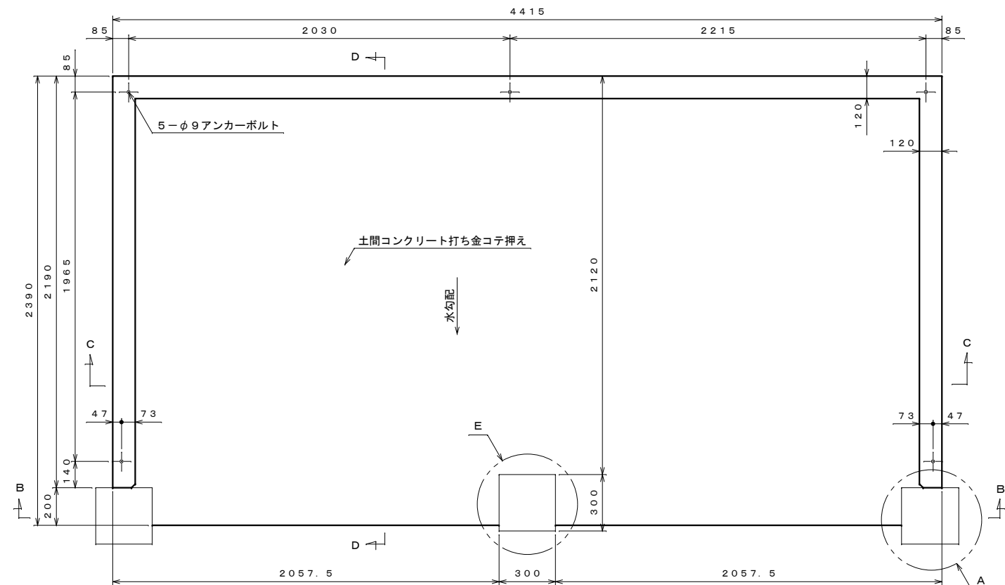
基礎伏せ図 S=1:20
