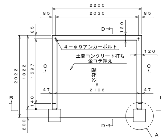
基礎伏図 S=1:40
