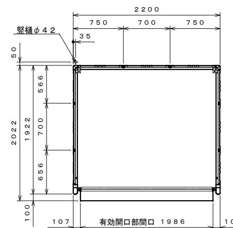
平面図 S=1:40
