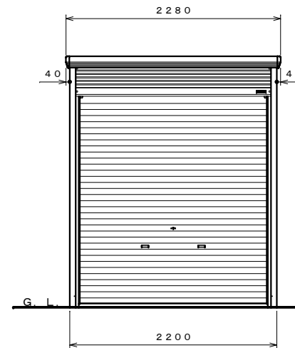
正面図 S=1:40
