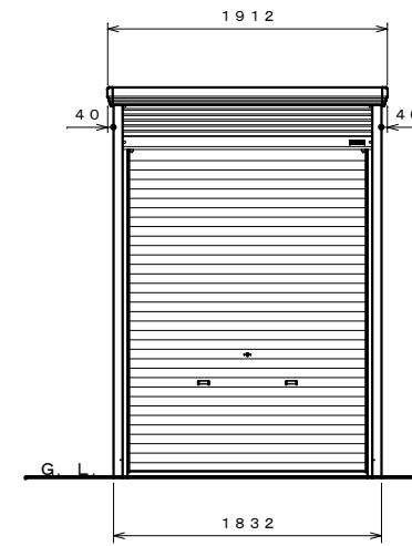
正面図 S=1:40
