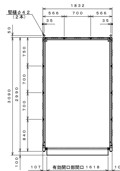
平面図 S=1:40
