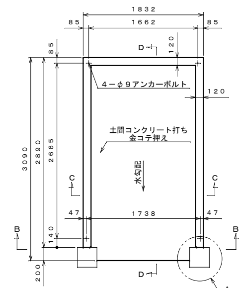
基礎伏せ図 S=1:40
