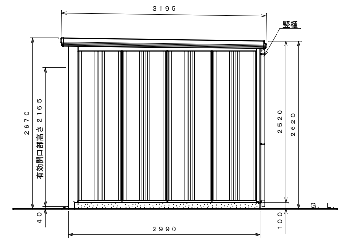
側面図 S=1:40
