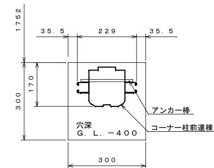
E部詳細図 S=1:10
