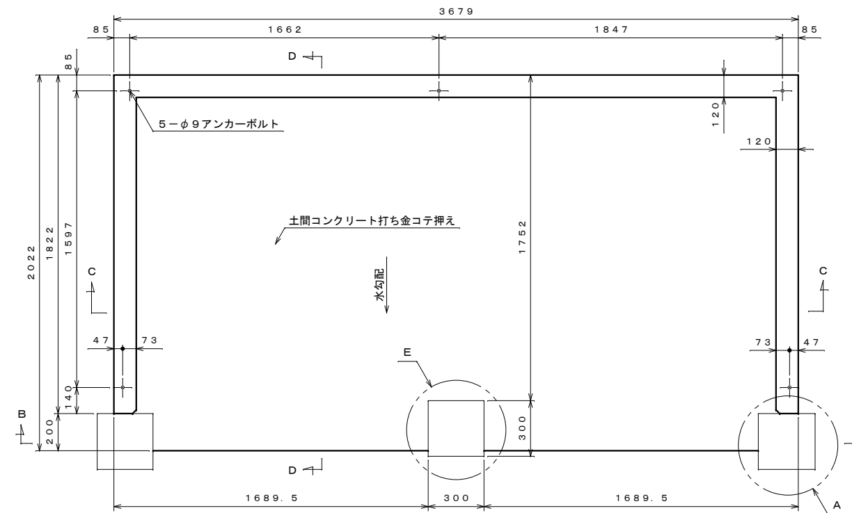
基礎伏せ図 S=1:20
