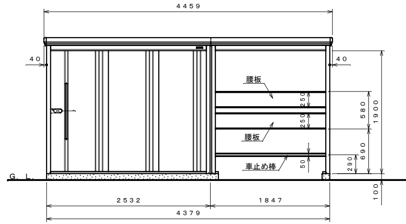
正面図 S=1:40
