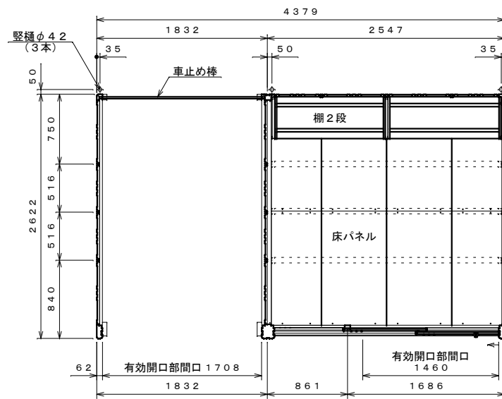
平面図 S=1:40
