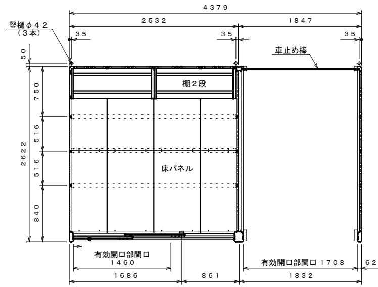
平面図 S=1:40
