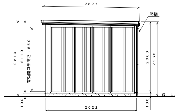
側面図 S=1:40
