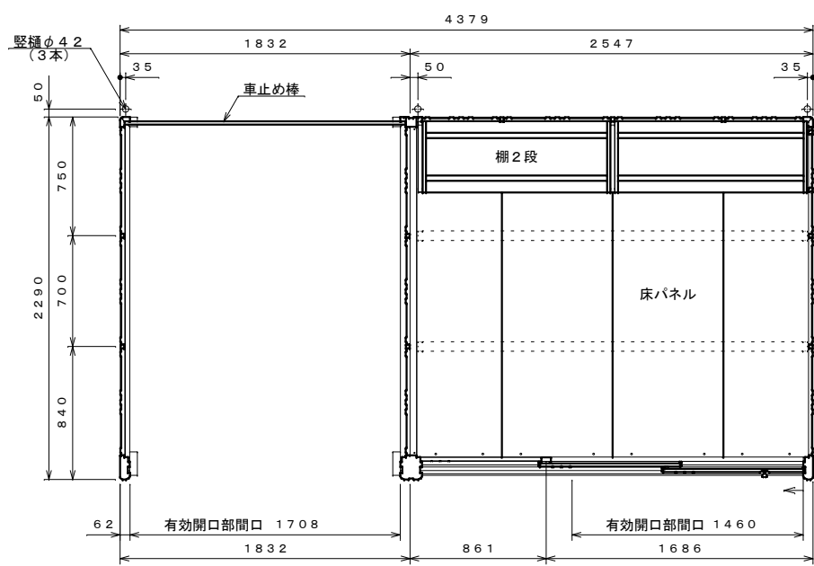
平面図 S=1:30
