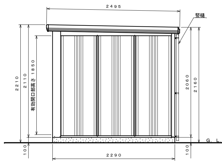
側面図 S=1:30
