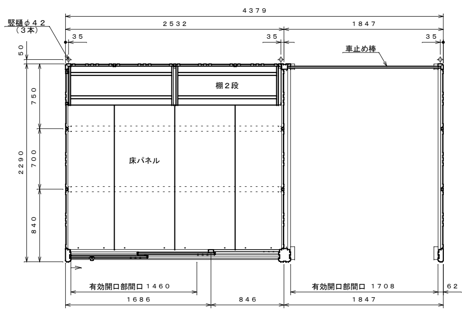
平面図 S=1:30
