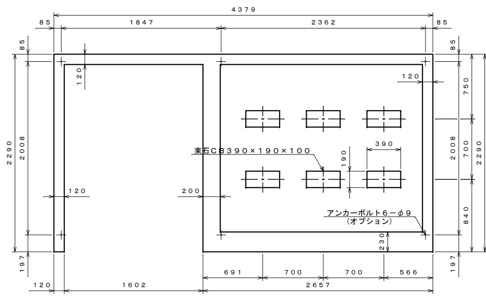
基礎伏せ図 S=1:30
