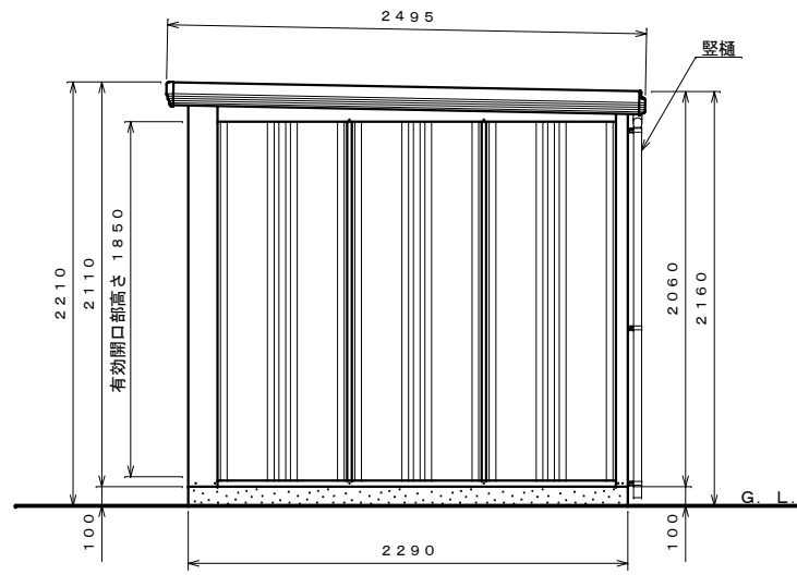
側面図 S=1:30
