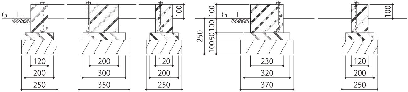
正面断面図
