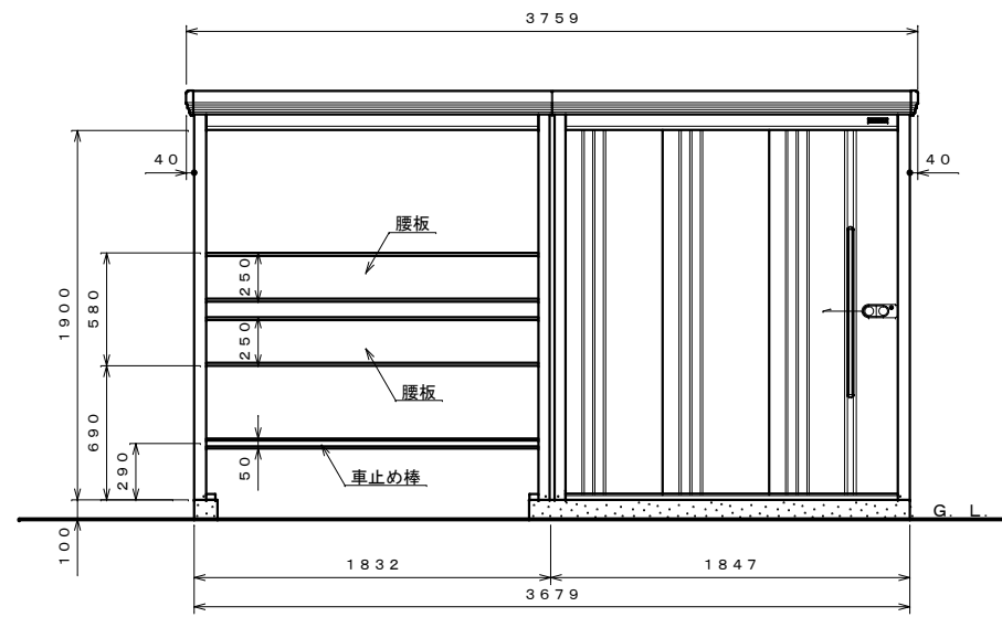
正面図 S=1:30
