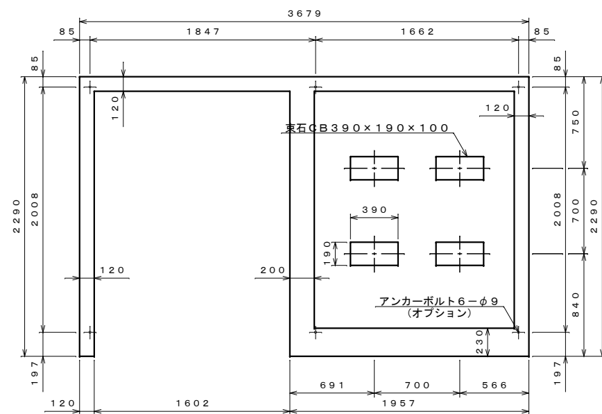
基礎伏せ図 S=1:30
