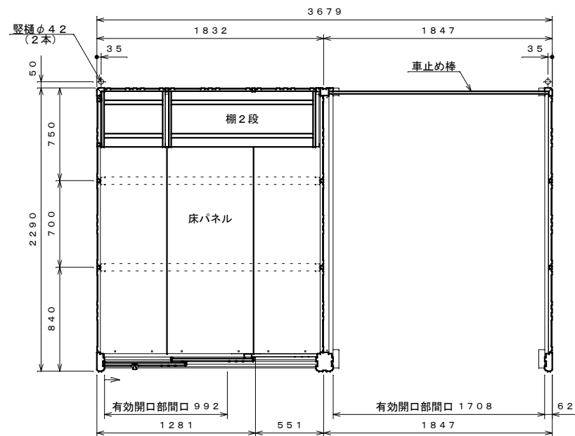
平面図 S=1:30
