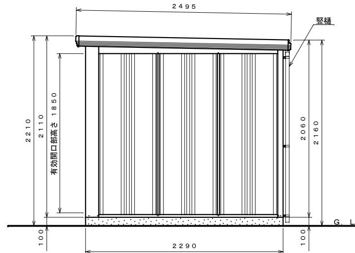
側面図 S=1:30
