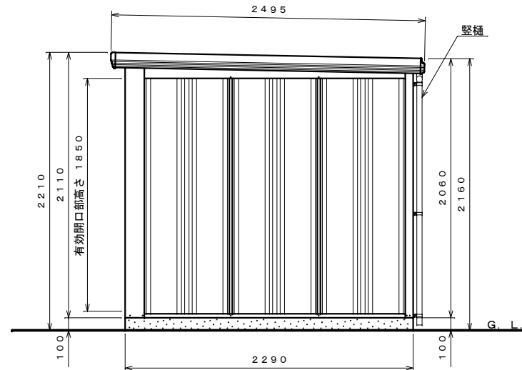
側面図 S=1:30
