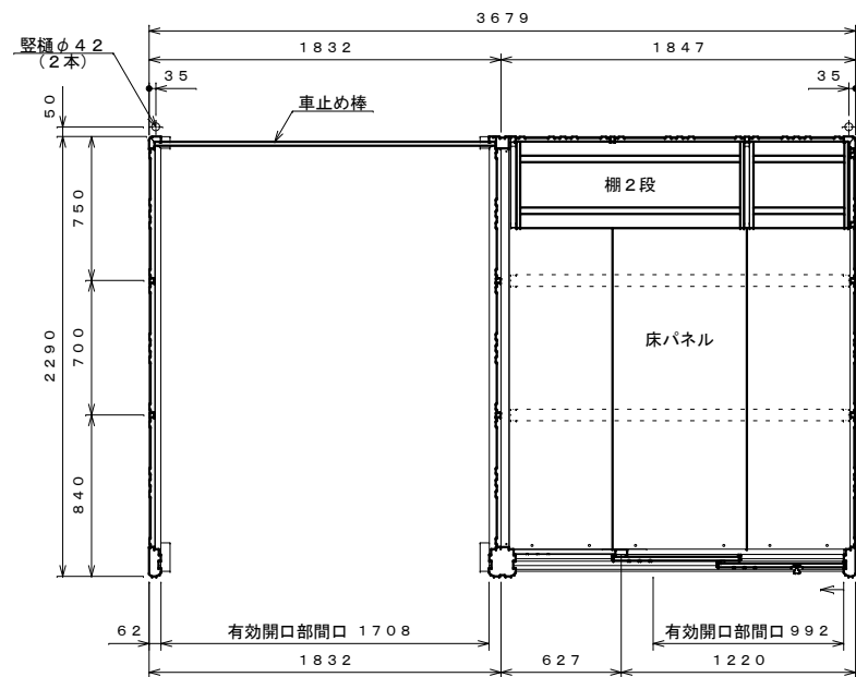
平面図 S=1:30
