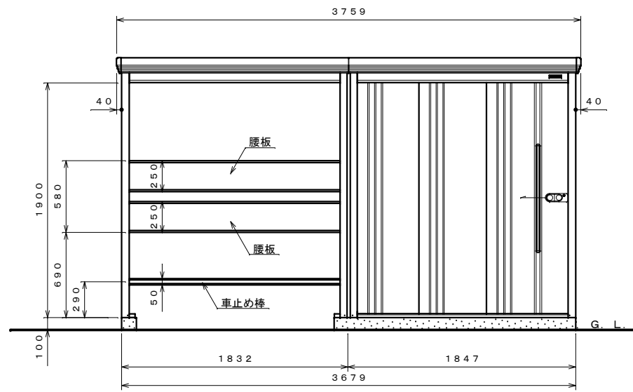
正面図 S=1:30
