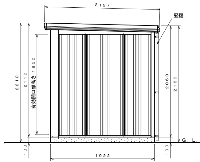
側面図 S=1:30
