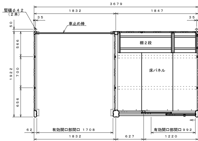
平面図 S=1:30
