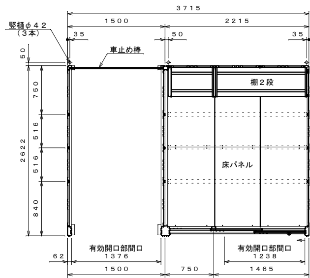
平面図 S=1:40
