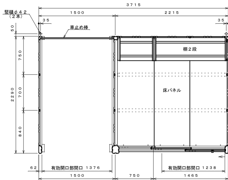
平面図 S=1:30
