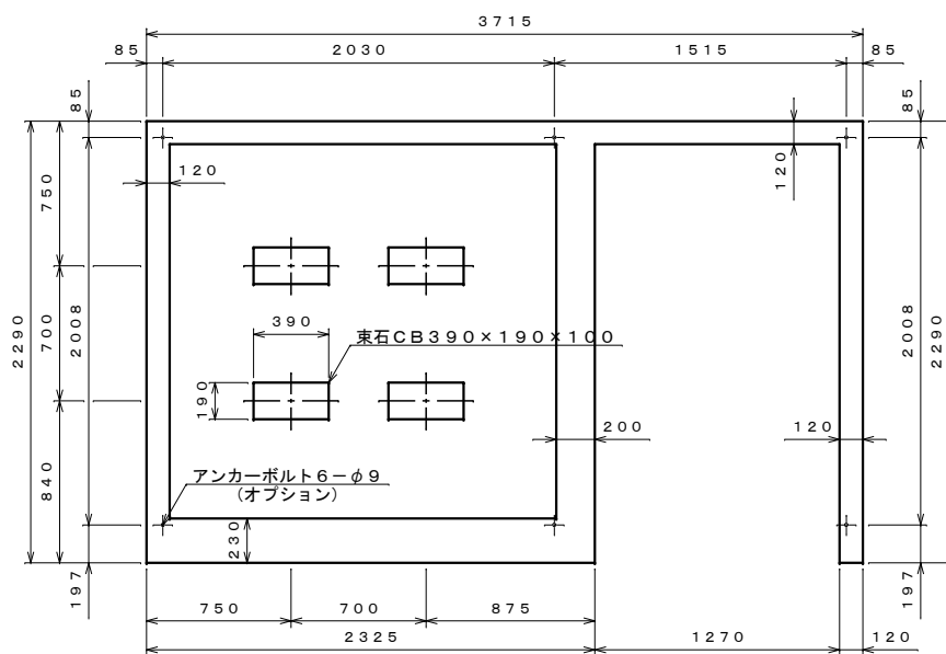
基礎伏図 S=1:30
