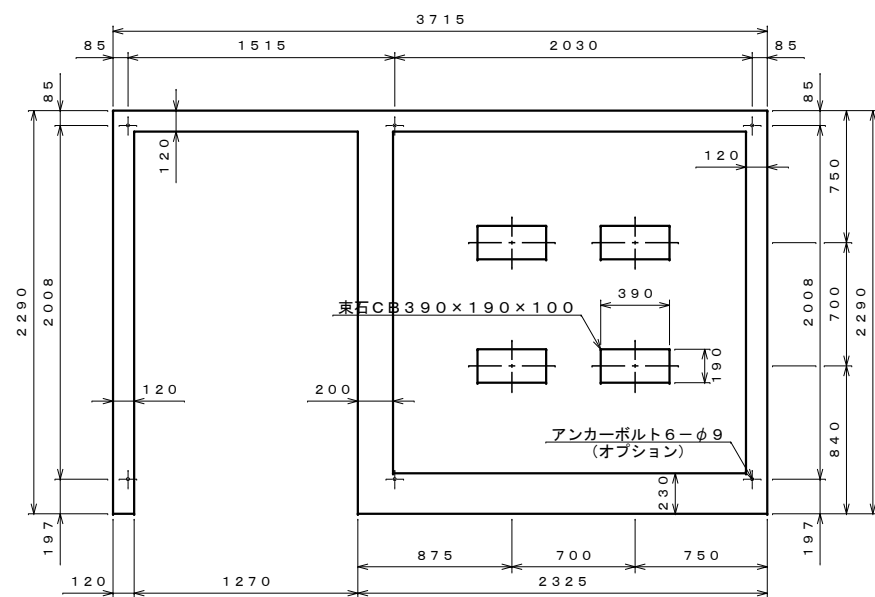
基礎伏図 S=1:30
