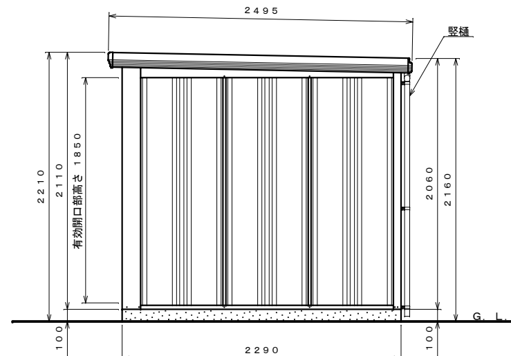
側面図 S=1:30
