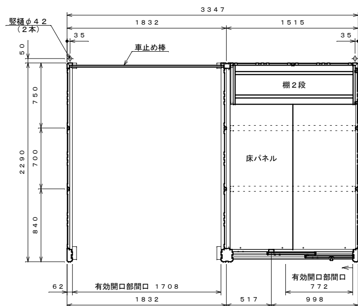
平面図 S=1:30
