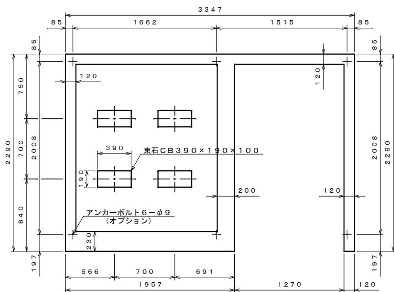
基礎伏せ図 S=1:30
