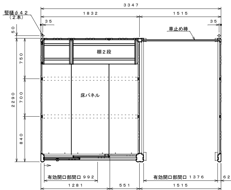
平面図 S=1:30
