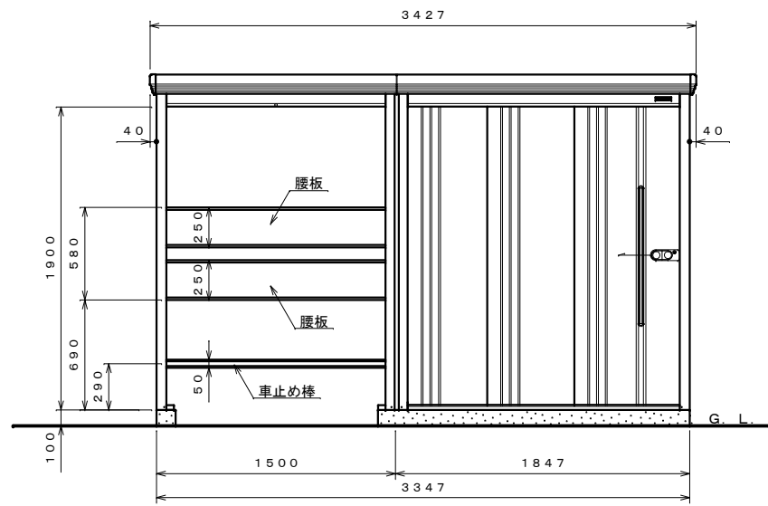
正面図 S=1:30
