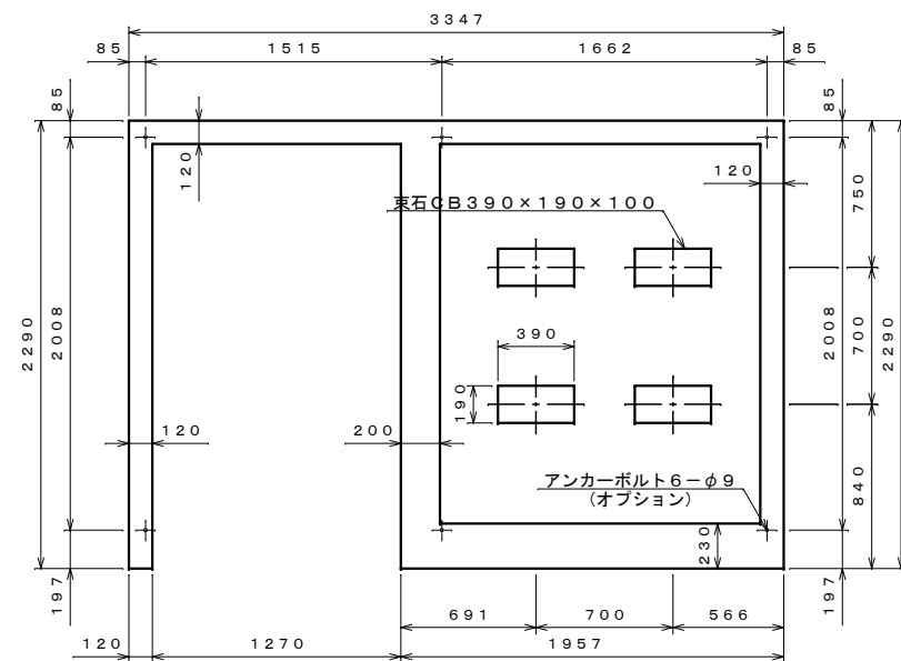
基礎伏せ図 S=1:30
