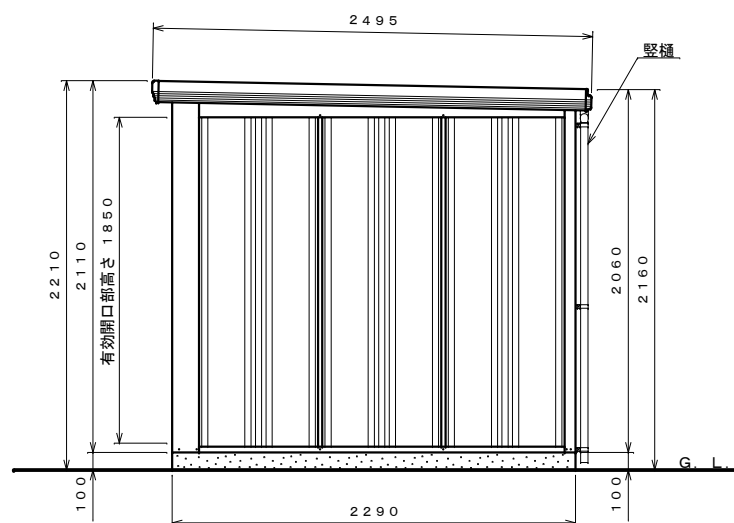
側面図 S=1:30
