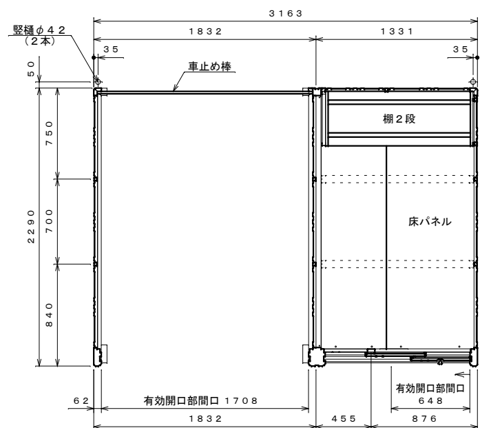
平面図 S=1:30
