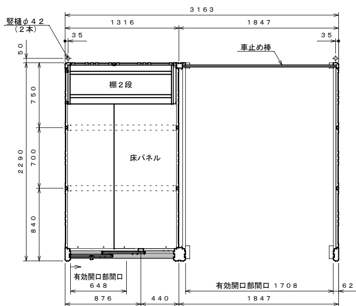
平面図 S=1:30
