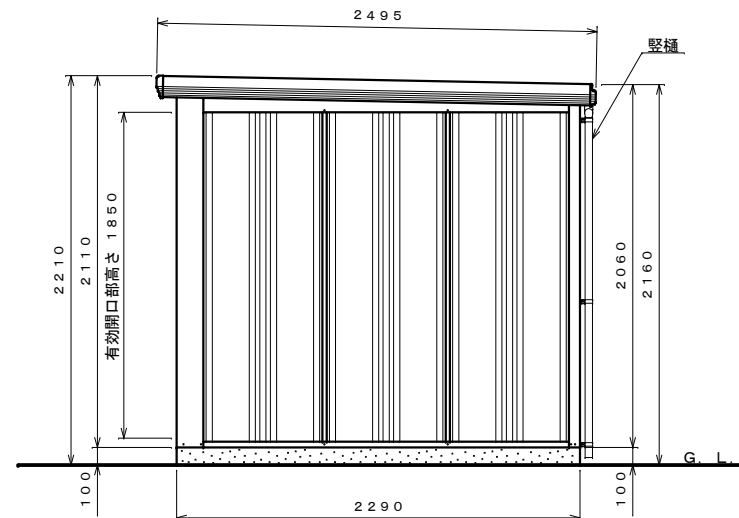
側面図 S=1:30
