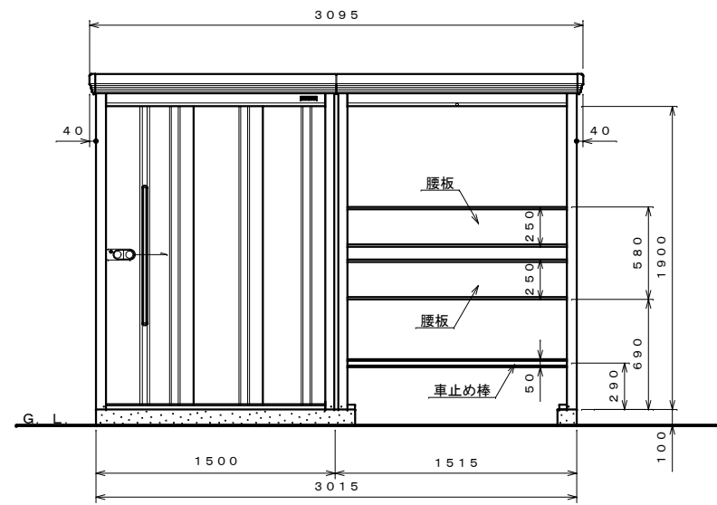
正面図 S=1:30
