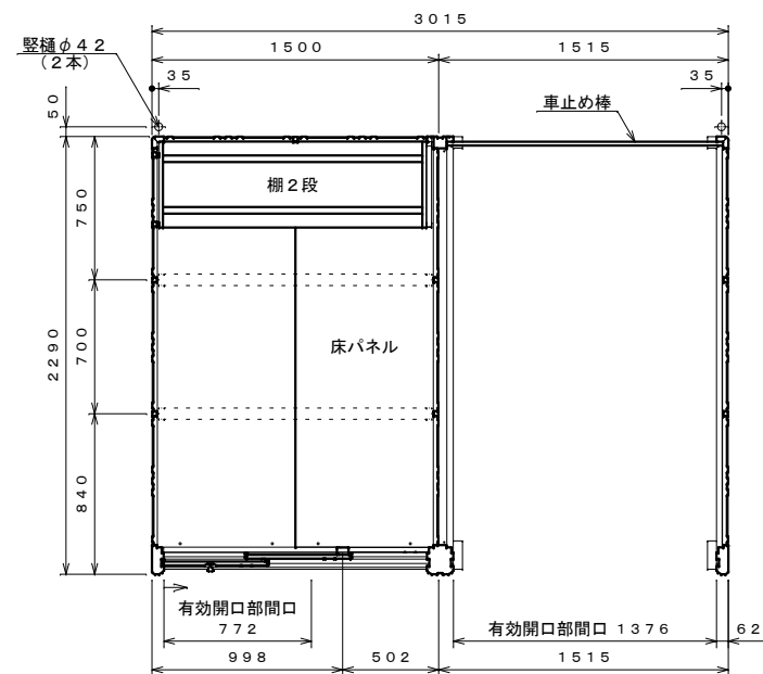
平面図 S=1:30
