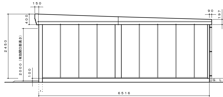
側面図 S=1:50
