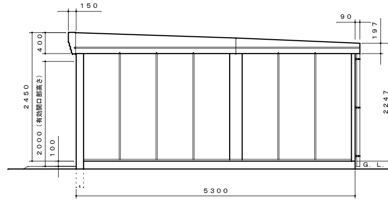
側面図 S=1:50
