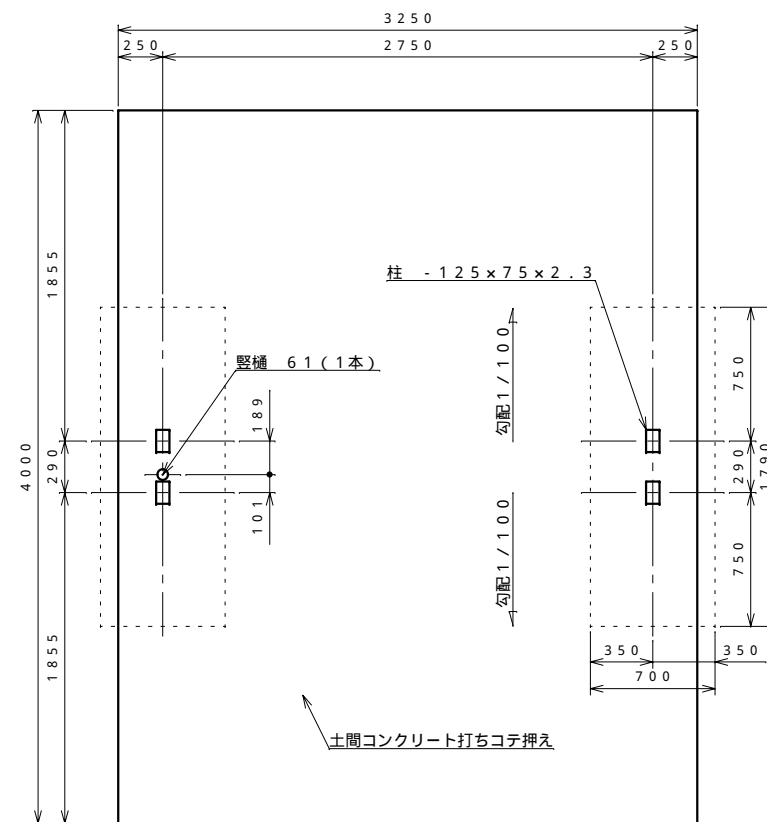
基礎伏せ図 S = 1 : 30
