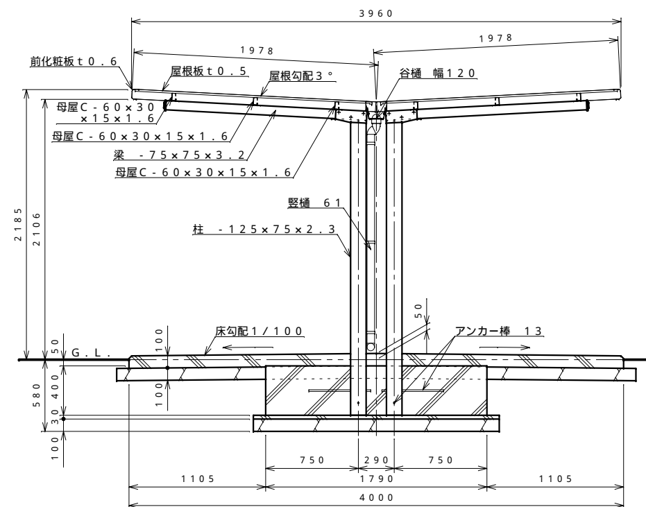
側面断面図 S = 1 : 30
