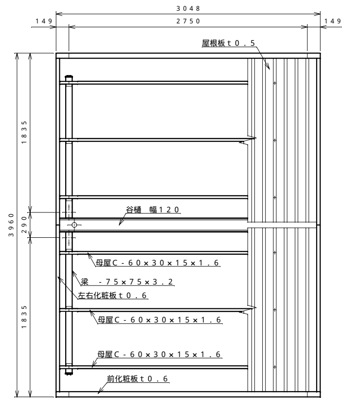
平面図 S = 1 : 30
