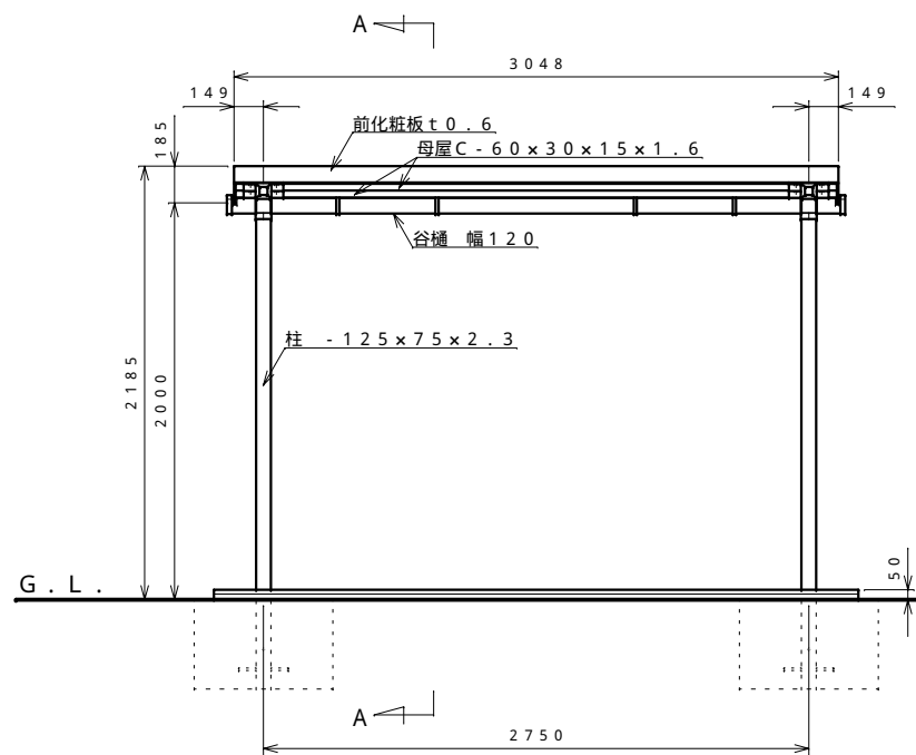
正面図 S = 1 : 30
