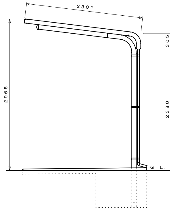
側面図 S=1:30
