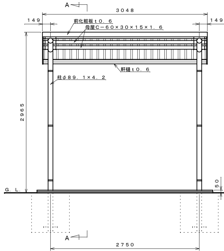
正面図 S=1:30
