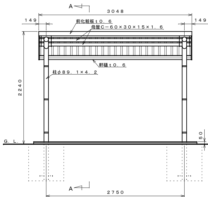
正面図 S=1:30
