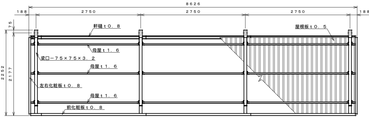
平面図 S=1:40
