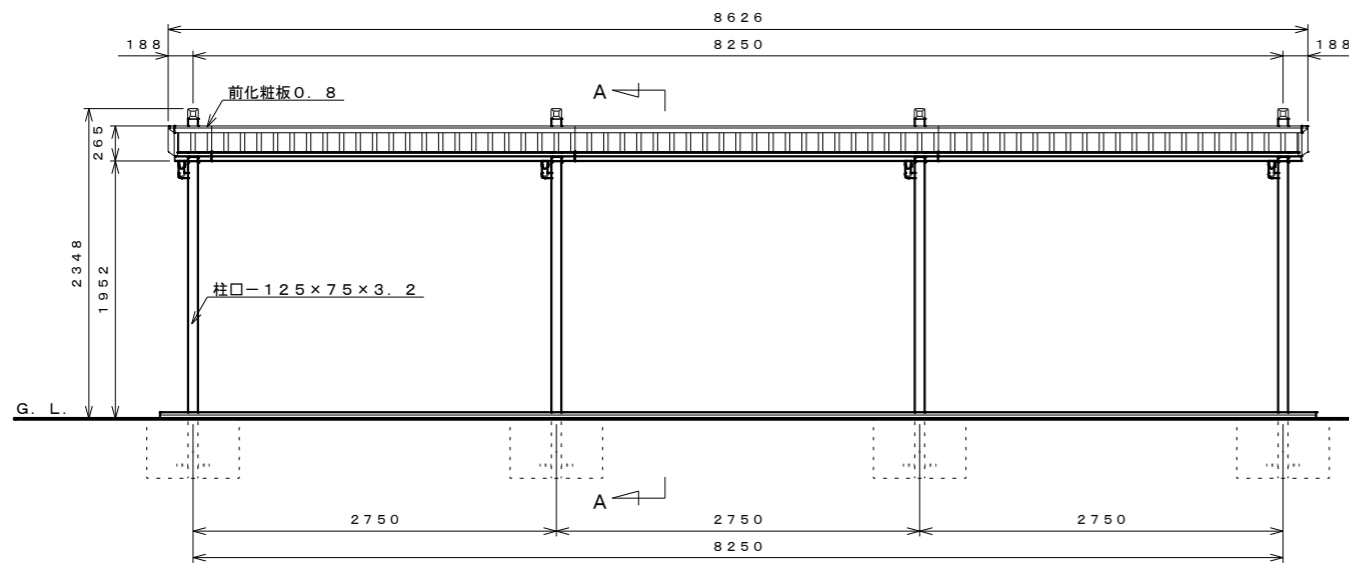
正面図 S=1:40
