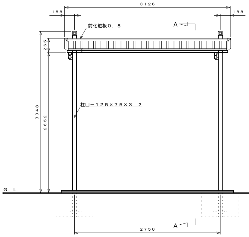
正面図 S=1:30
