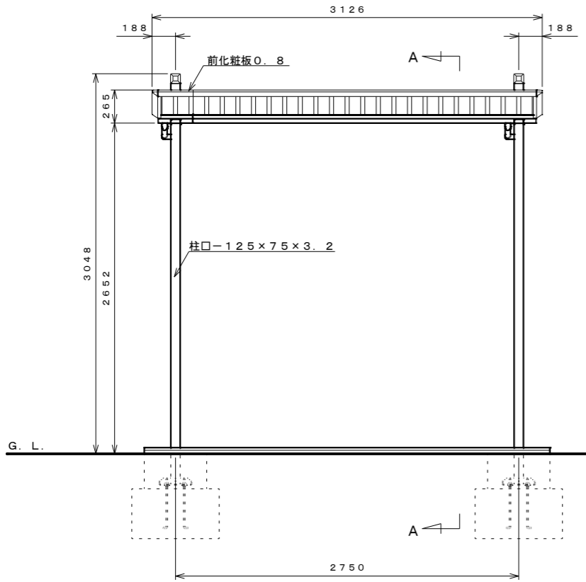
正面図 S=1:30
