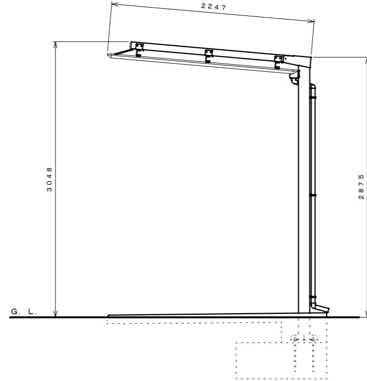
側面図 S=1:30
