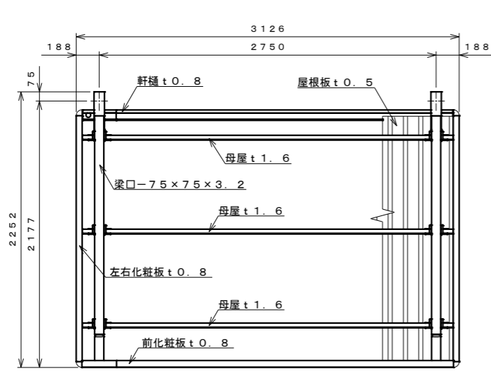
平面図 S=1:30
