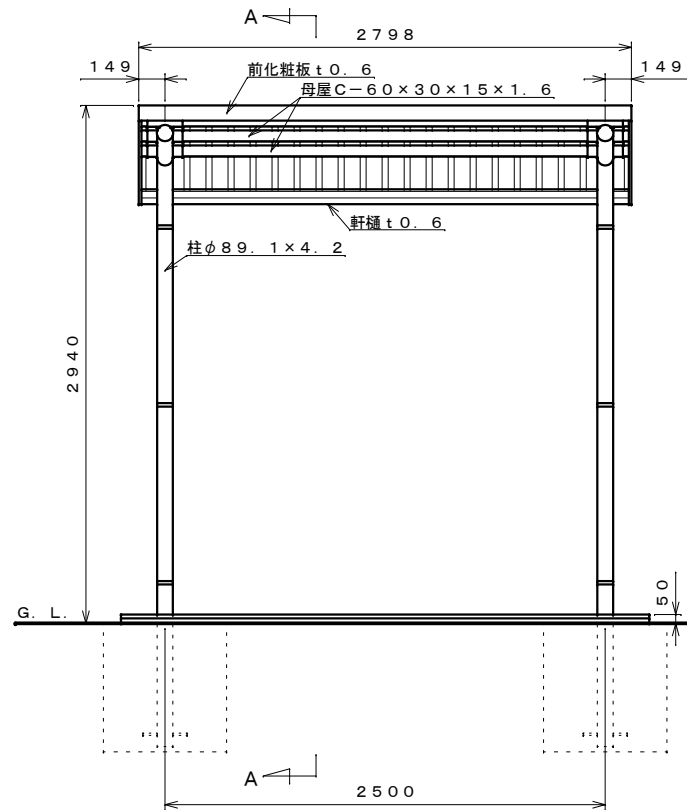
正面図 S=1:30
