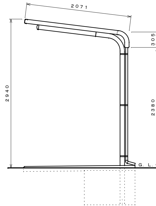
側面図 S=1:30
