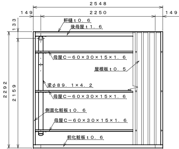
平面図 S=1:30
