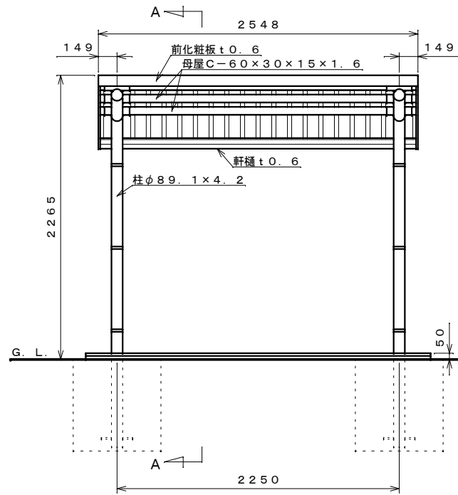
正面図 S=1:30
