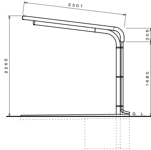
側面図 S=1:30
