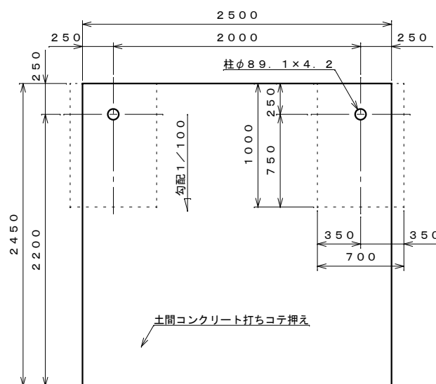
基礎伏せ図 S=1:30 (注: この基礎は標準を示しています。現場の実情に合わせて、ご設計下さい。)
