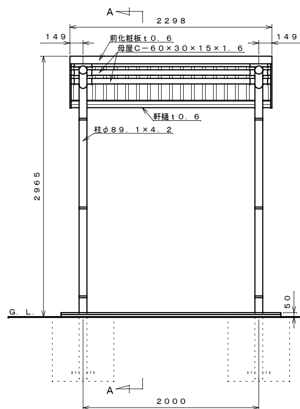
正面図 S=1:30
