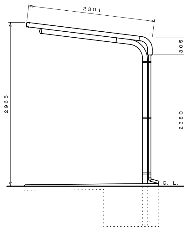
側面図 S=1:30
