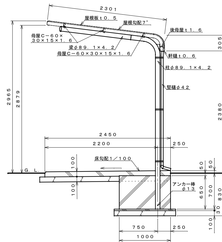
A-A断面図 S=1:30 コンクリート強度: Fc 21 N/mm 2 以上
