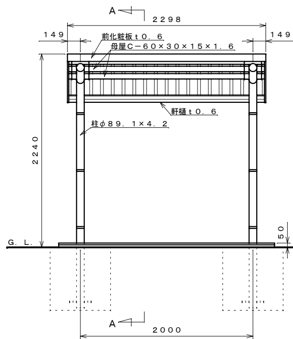
正面図 S=1:30
