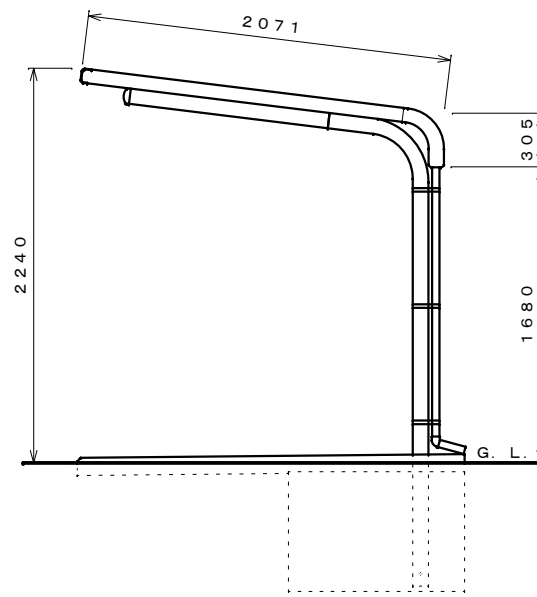
側面図 S=1:30
