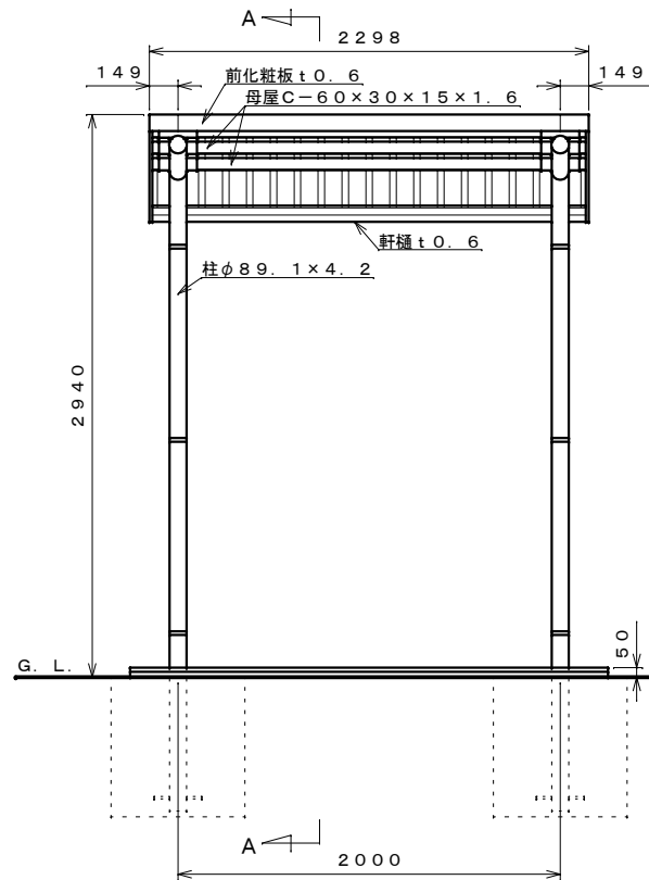
正面図 S=1:30
