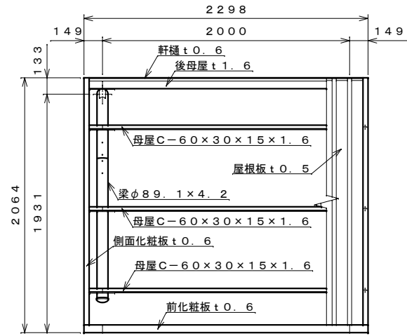
平面図 S=1:30
