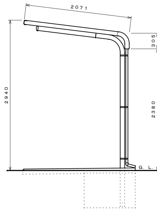
側面図 S=1:30
