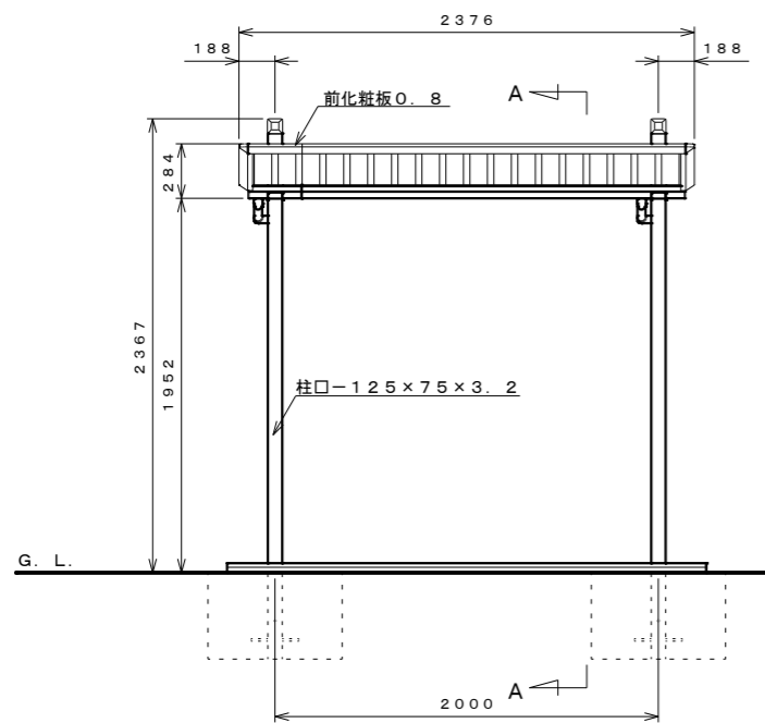
正面図 S=1:30
