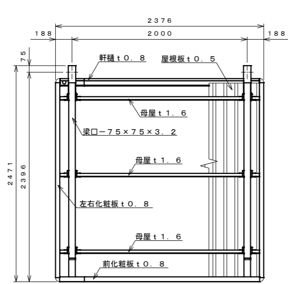
平面図 S=1:30
