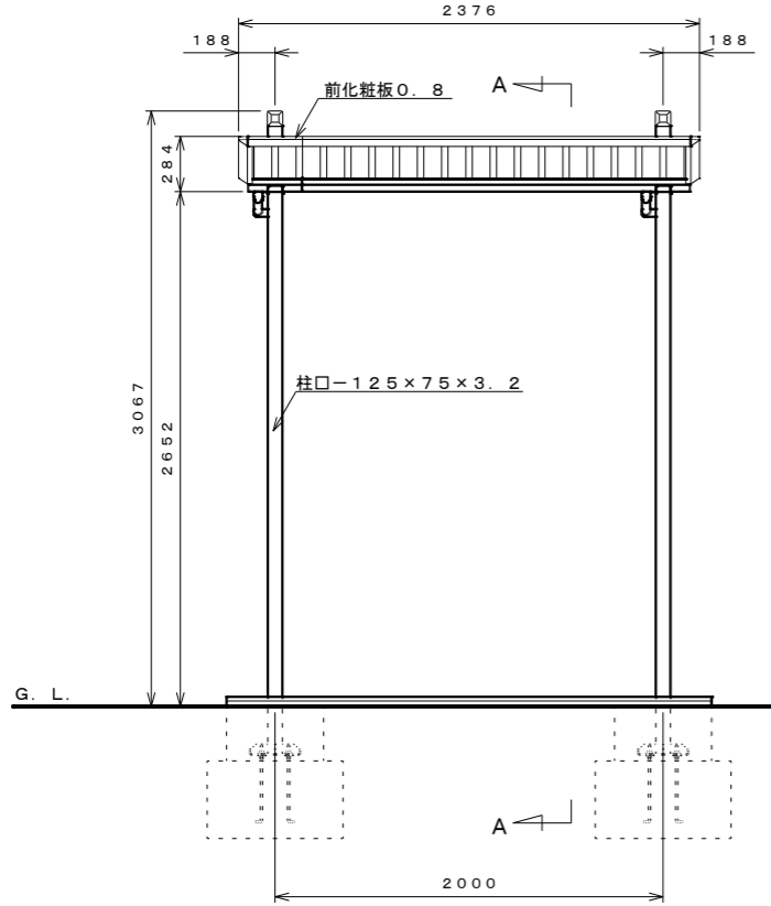
正面図 S=1:30
