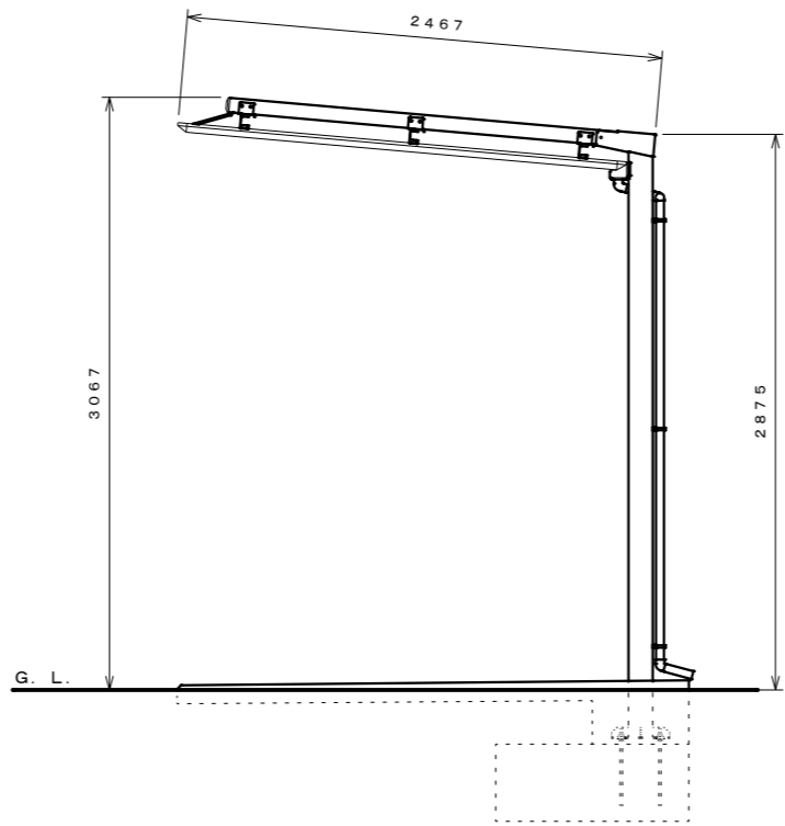
側面図 S=1:30
