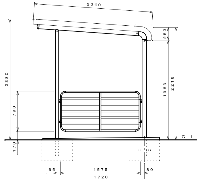
側面図 S=1:30
