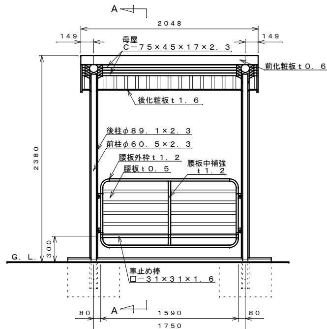
正面図 S=1:30
