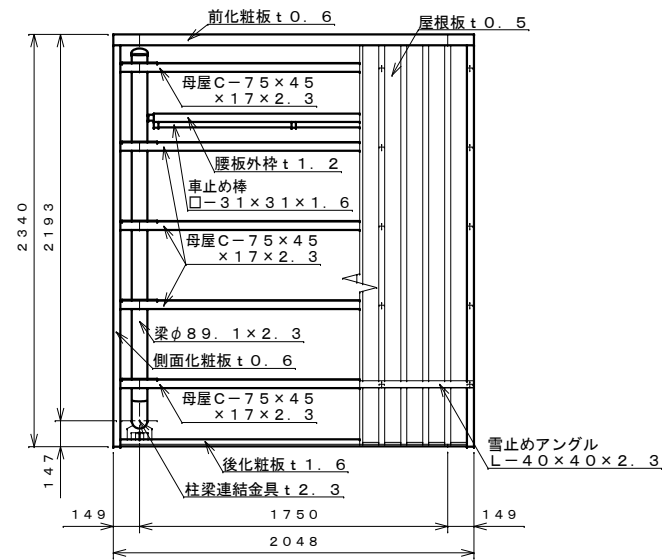
平面図 S=1:30
