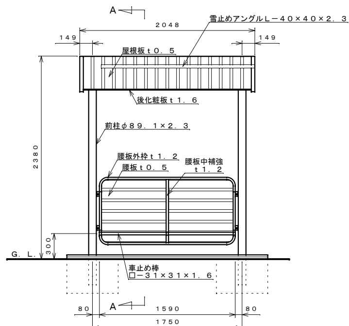
正面図 S=1:30
