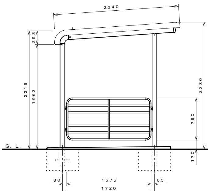
側面図 S=1:30
