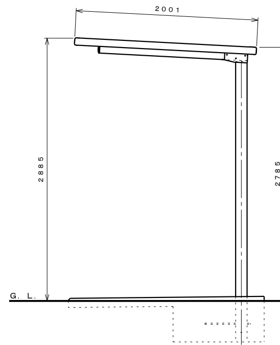
側面図 S=1:30
