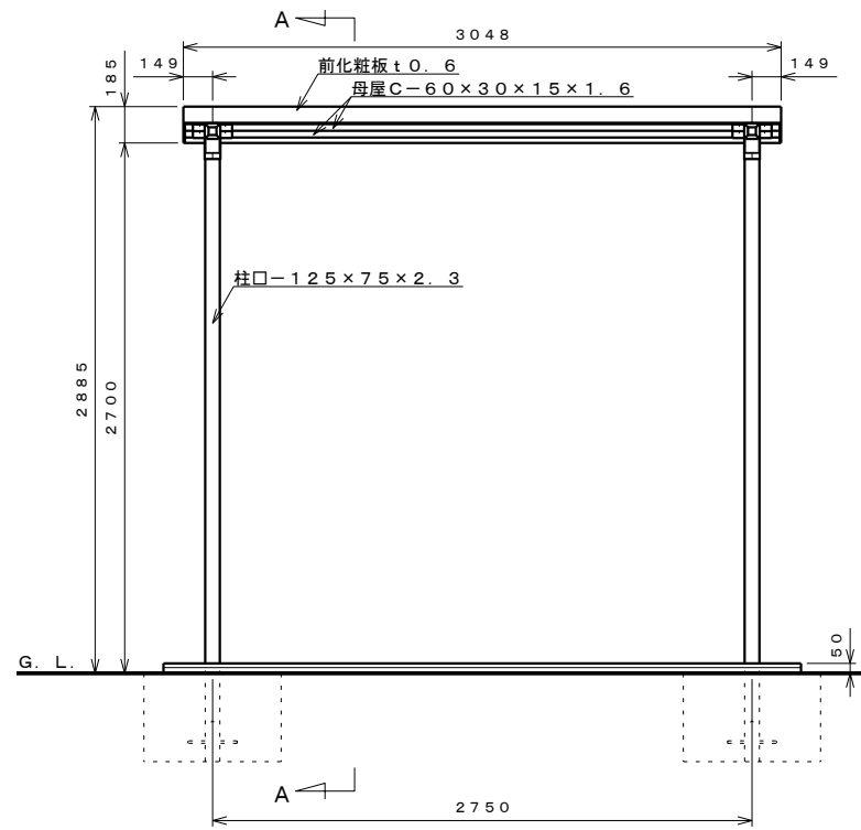
正面図 S=1:30
