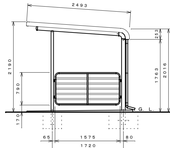
側面図 S=1:40
