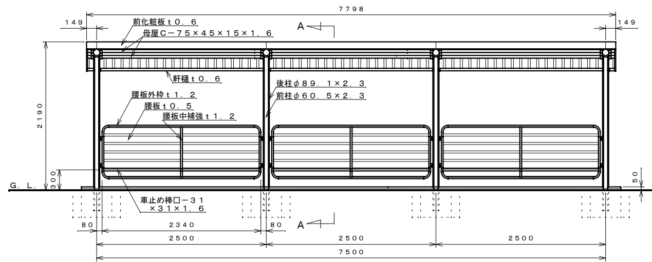
正面図 S=1:40
