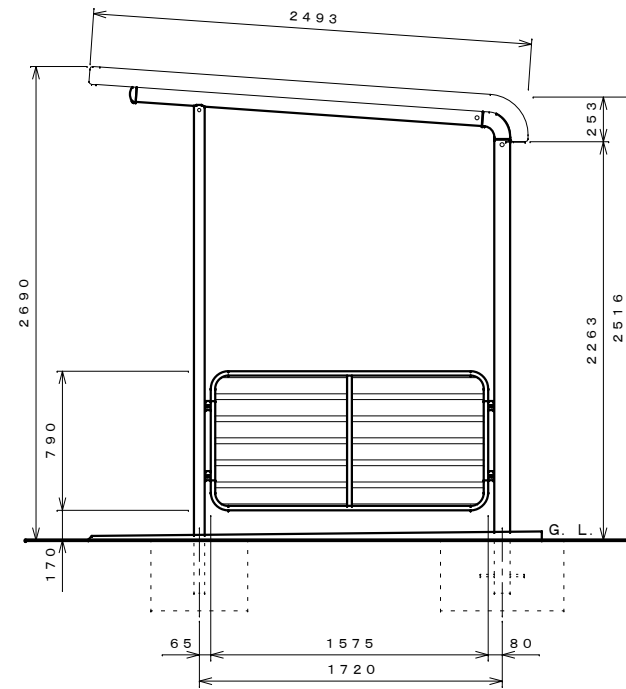
側面図 S=1:30
