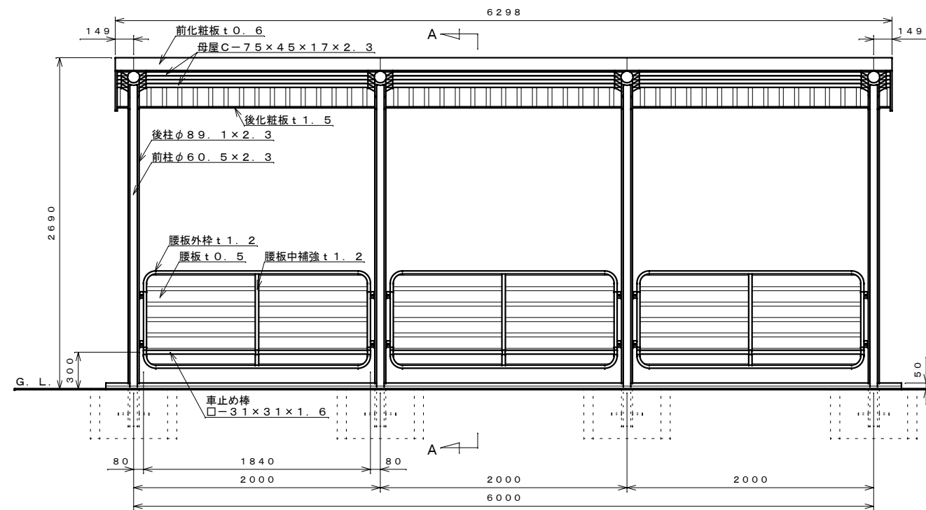
正面図 S=1:30
