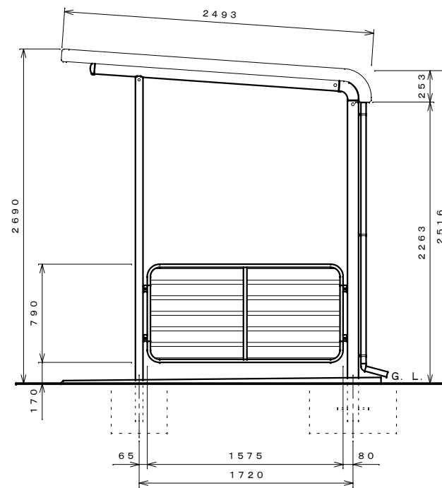
側面図 S=1:30
