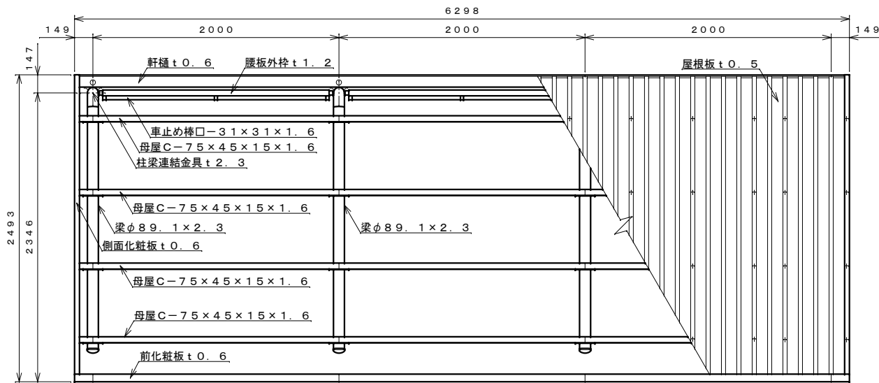
平面図 S=1:30
