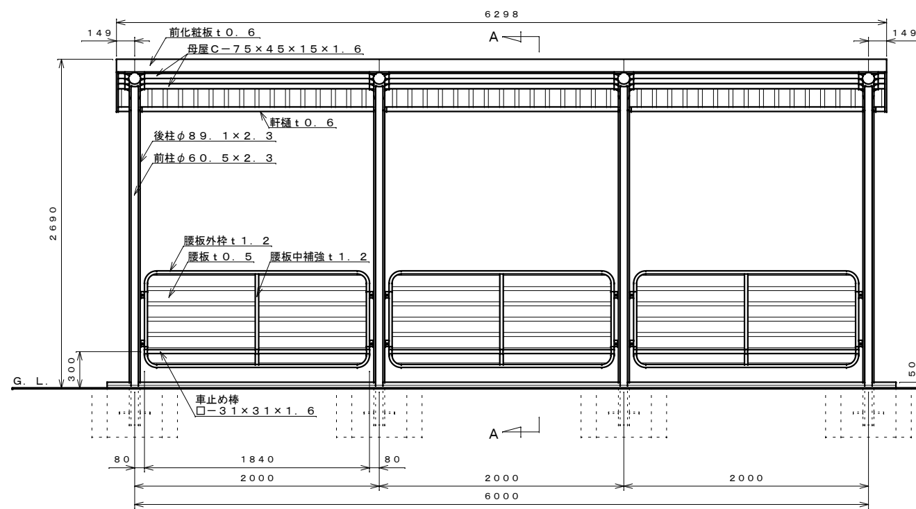
正面図 S=1:30
