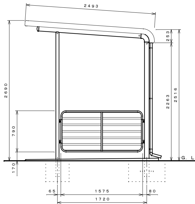
側面図 S=1:30
