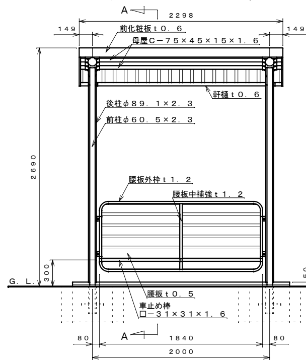
正面図 S=1:30
