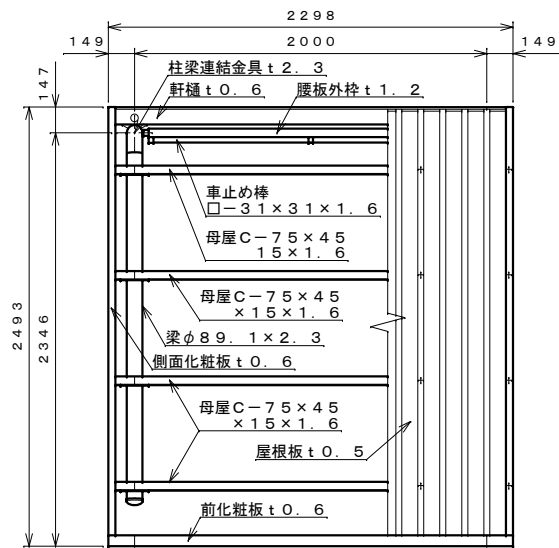
平面図 S=1:30
