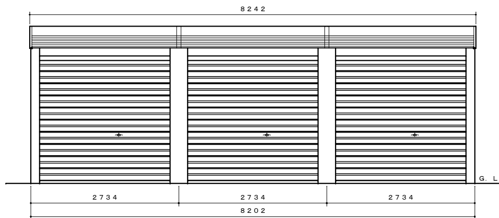
正面図 S=1:50
