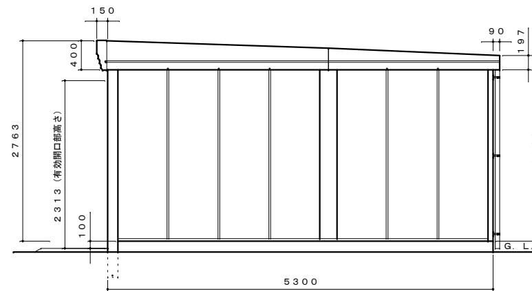
側面図 S=1:50
