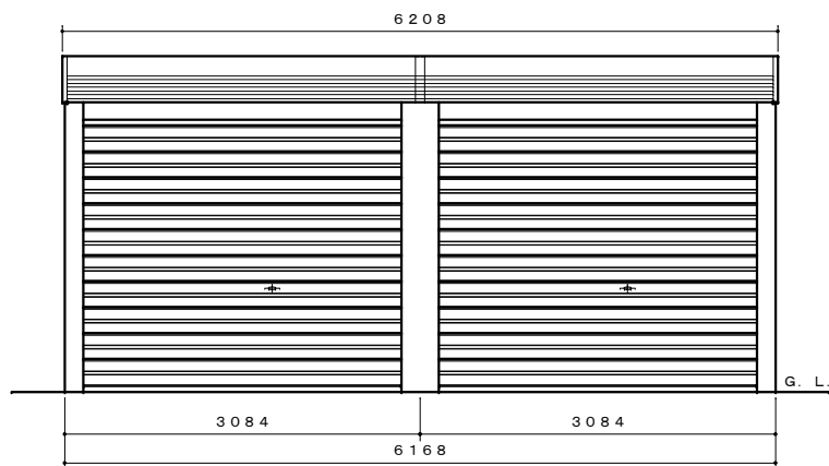
正面図 S=1:50
