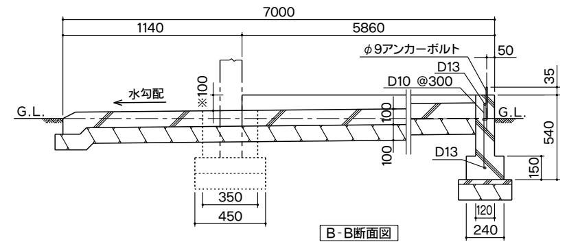
B-B断面図
