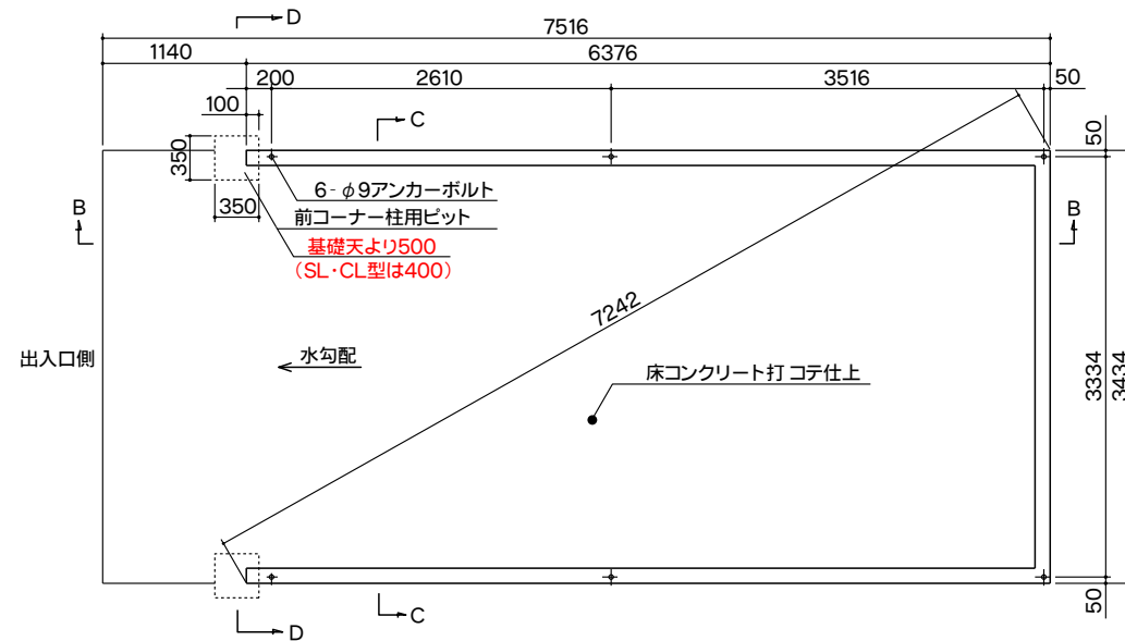
基礎伏せ図
