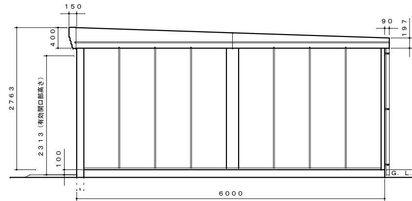
側面図 S=1:50
