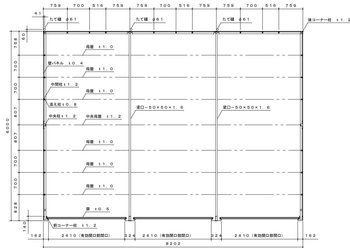
平面図 S=1:50
