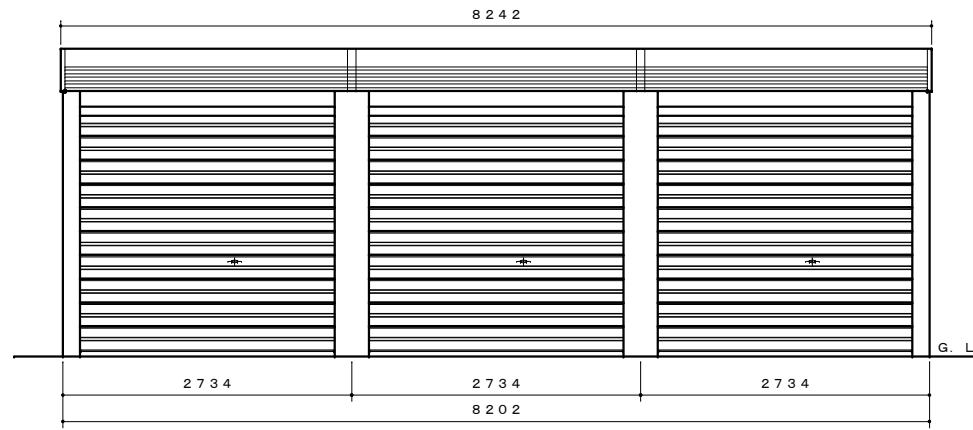
正面図 S=1:50
