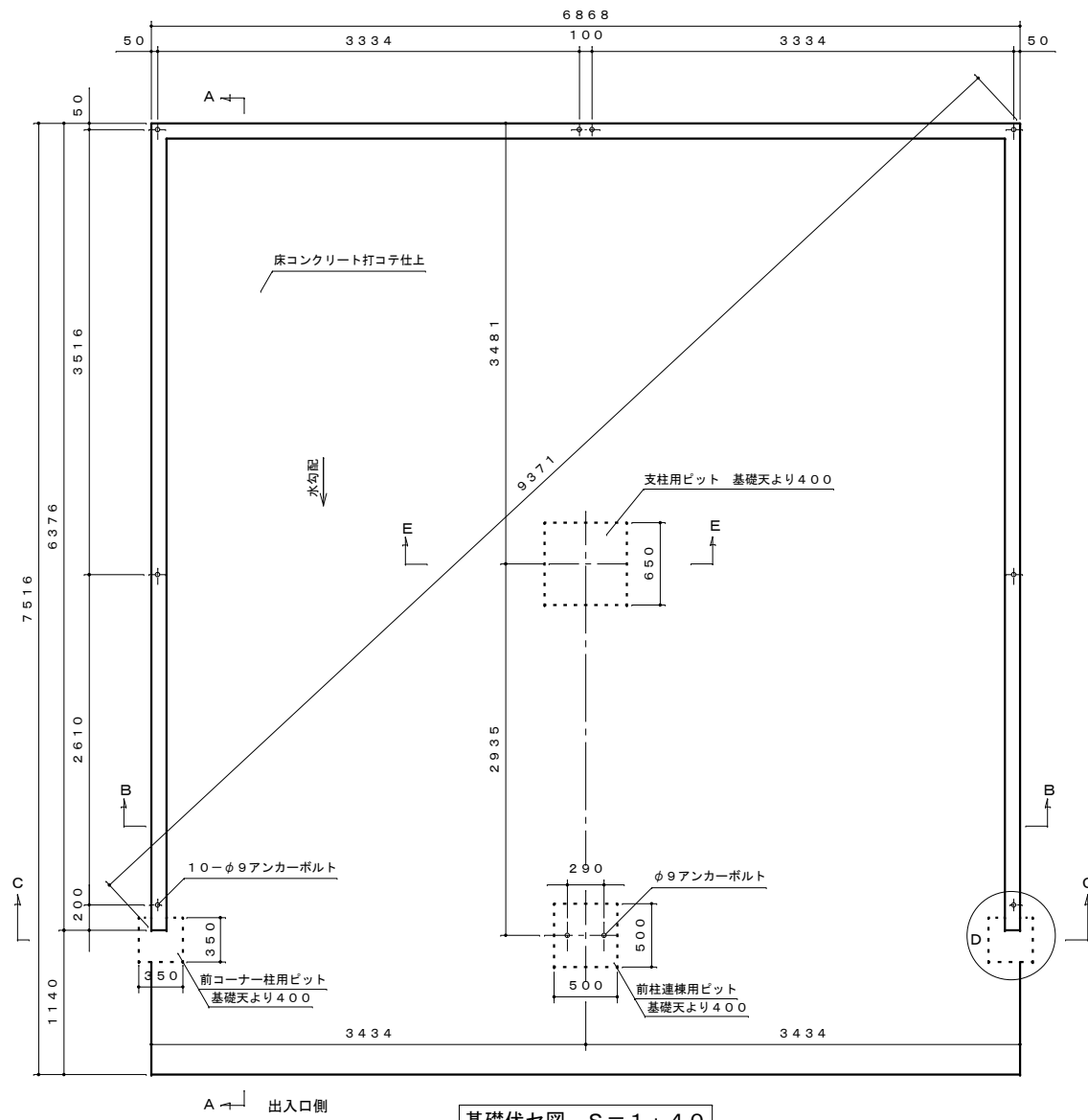
基礎伏せ図 S=1:40
